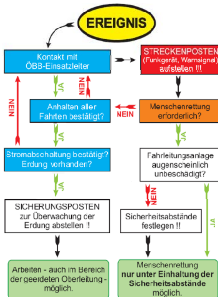
Abbildung 5.02 – Bedingungen für den Einsatz im Gleisbereich
