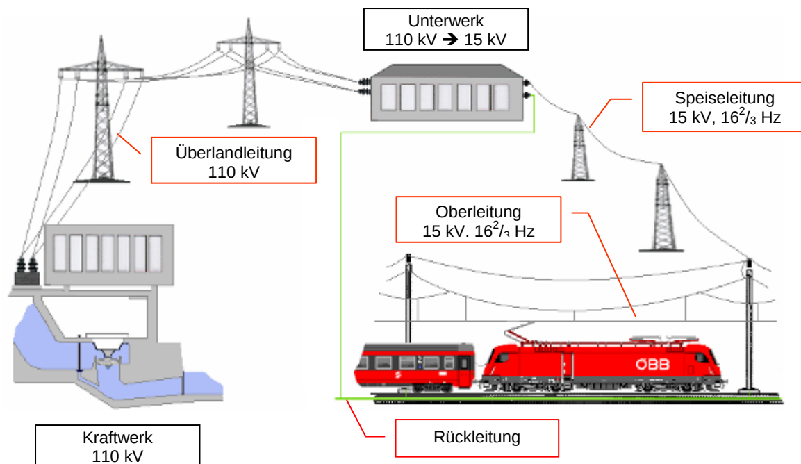
Abbildung 8.01 – Der Weg des Stromes vom Kraftwerk zum Triebfahrzeug
