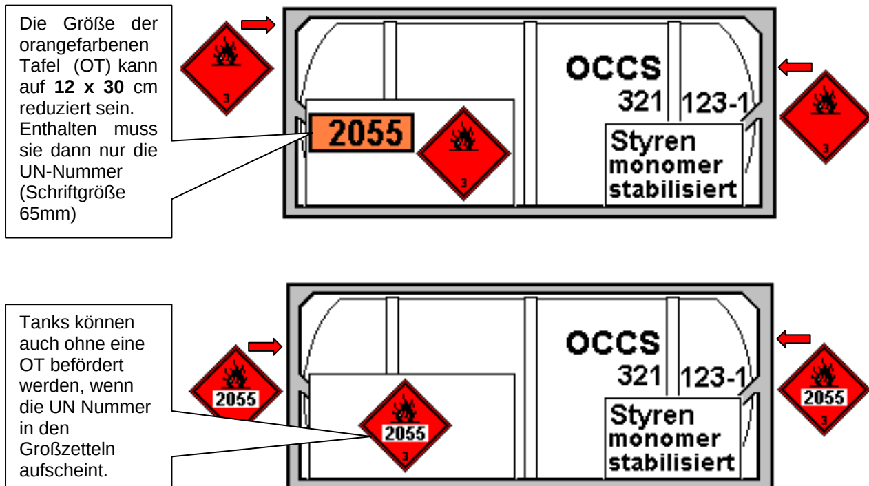
Abbildung 9.18 – Abweichende Kennzeichnung zum Seeverkehr
