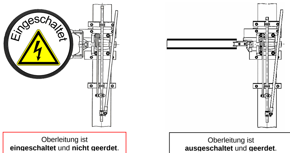
Abbildung 8.12 – Schaltzeiger des Ladegleisschalters - neu
