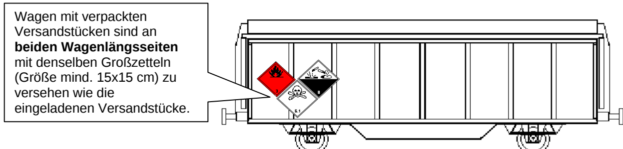
Abbildung 9.08 – Kennzeichnung: Gefahrgutversandstücke
