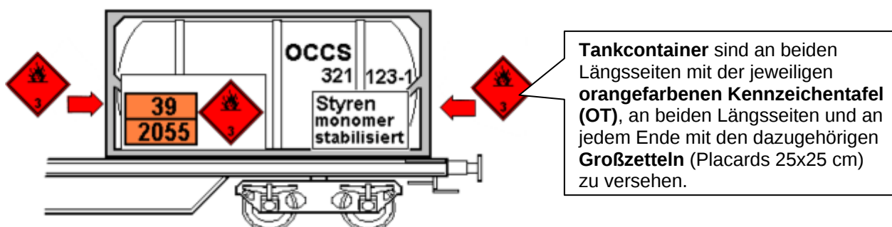
Abbildung 9.06 – Kennzeichnung: Tankcontainer mit Gefahrgütern
