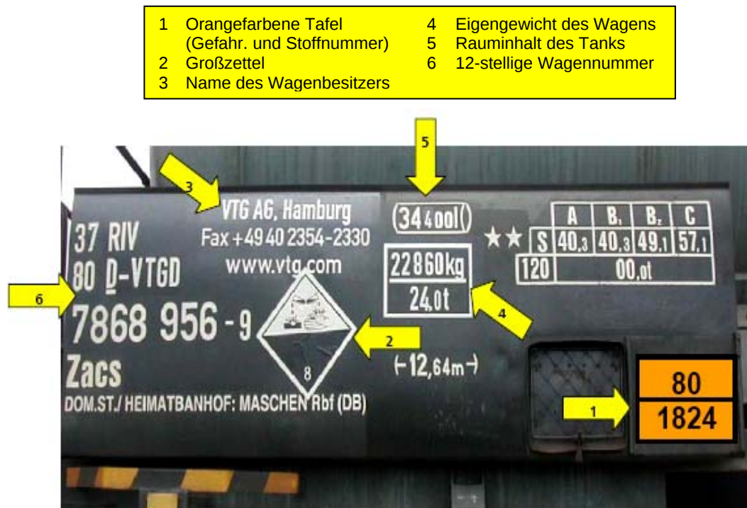
Abbildung 9.01 – Aufschriften an einem Gefahrgutkesselwagen
