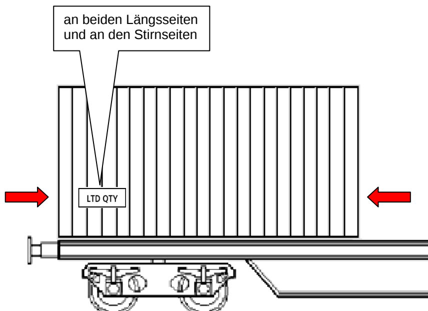
Abbildung 9.20 – Begrenzte Beförderung von Gefahrgütern in Containern
