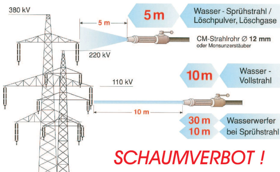
Abbildung 8.07 – Sicherheitsabstände bei Löscharbeiten
