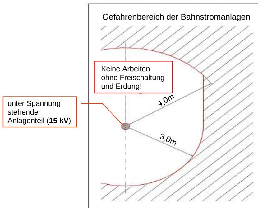
Abbildung 8.03 – Gefahrenbereich der Bahnstromanlagen
