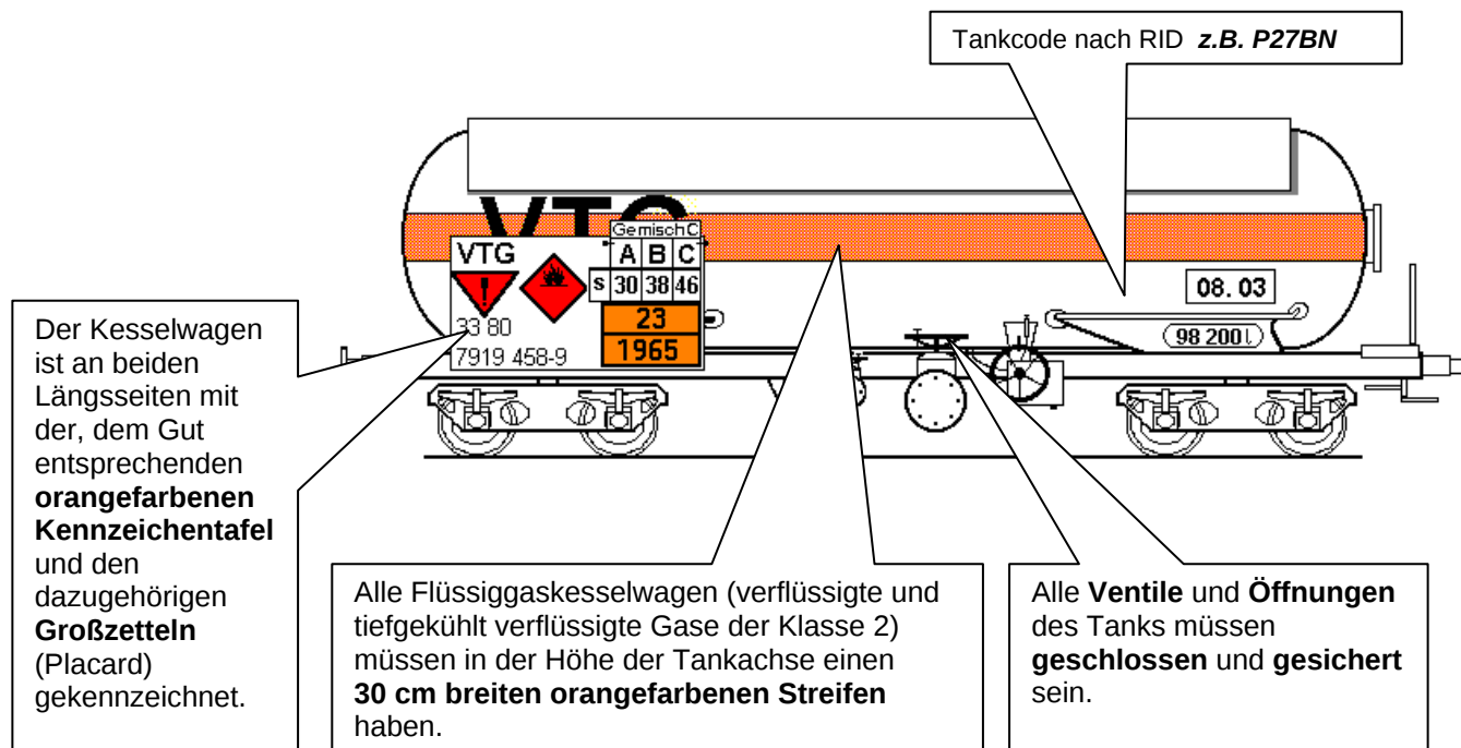
Abbildung 9.04 – Kennzeichnung: Flüssiggaskesselwagen
