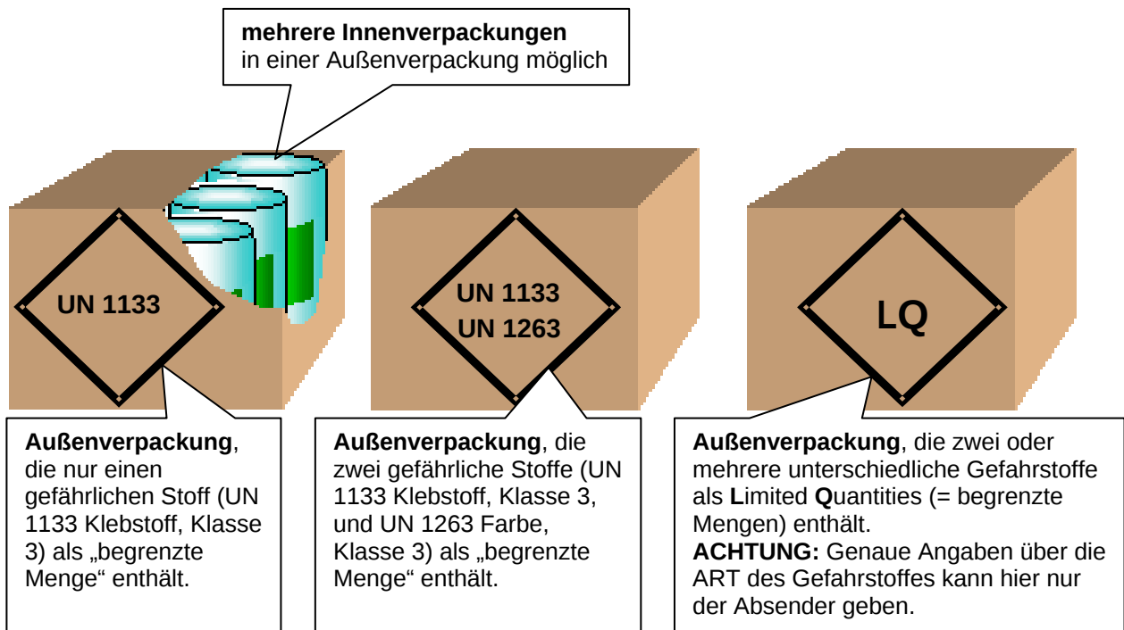
Abbildung 9.17 – Kennzeichnung an Verpackungen
