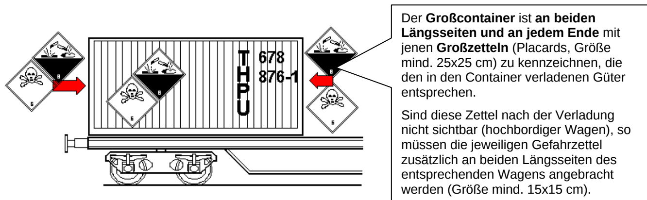
Abbildung 9.11 – Kennzeichnung: Großcontainer mit Gefahrgütern
