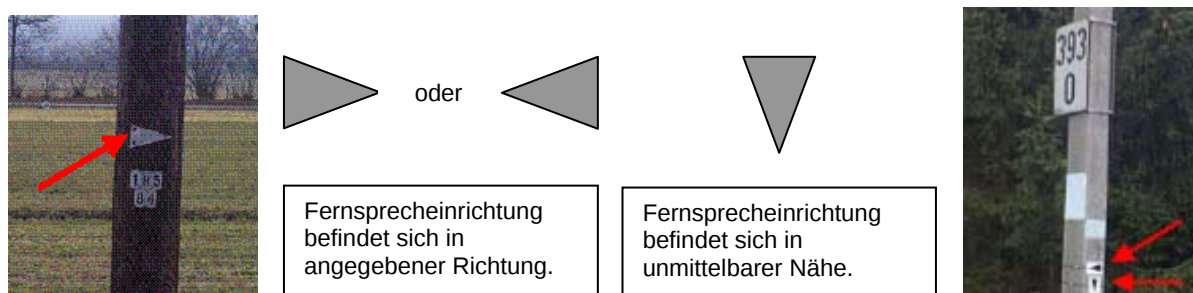
Abbildung 6.09 – Auffinden von Fernsprechstellen
