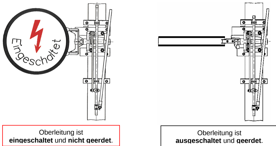
Abbildung 8.11 – Schaltzeiger des Ladegleisschalters - aktuell
