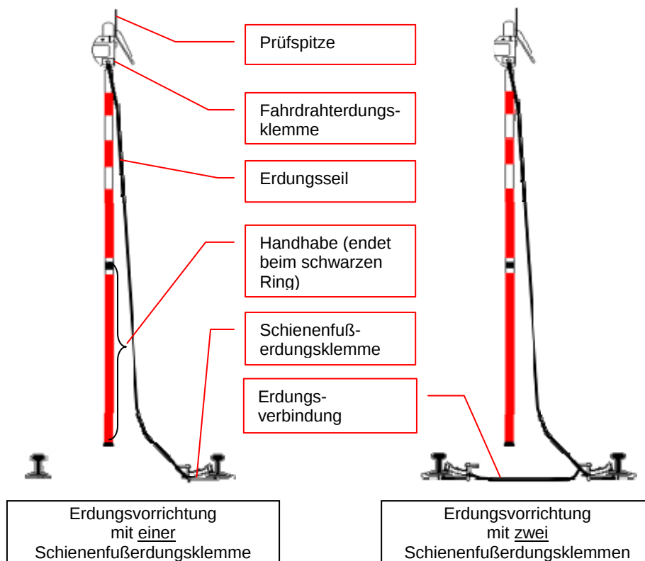
Abbildung 8.08 – Bestandteile einer Erdungsvorrichtung
