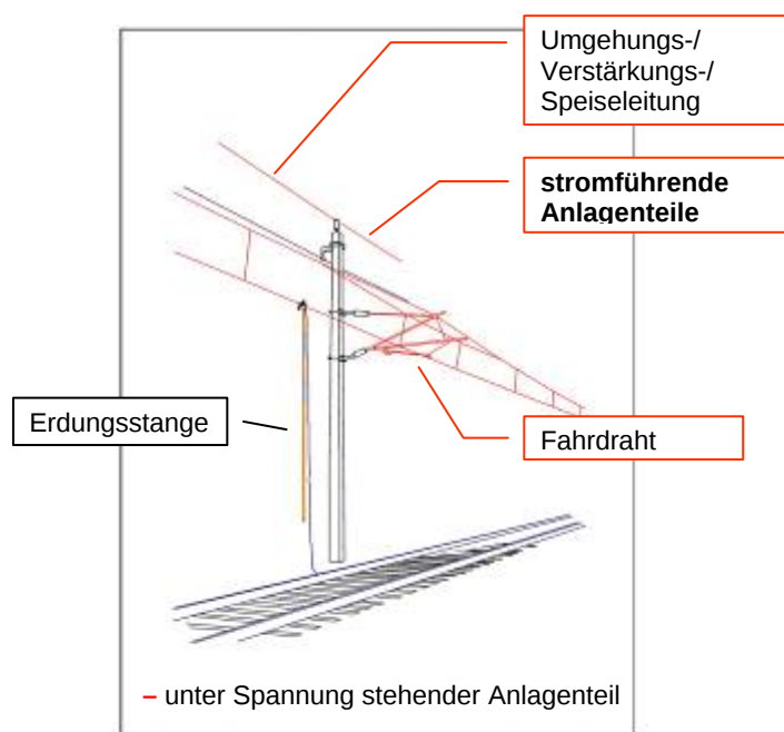
Abbildung 8.02 – Die Oberleitungsanlage
