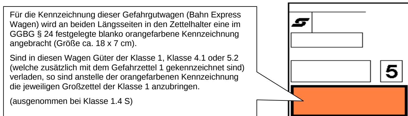
Abbildung 9.10 – Kennzeichnung: Wagen mit Gefahrgutversandstücke
