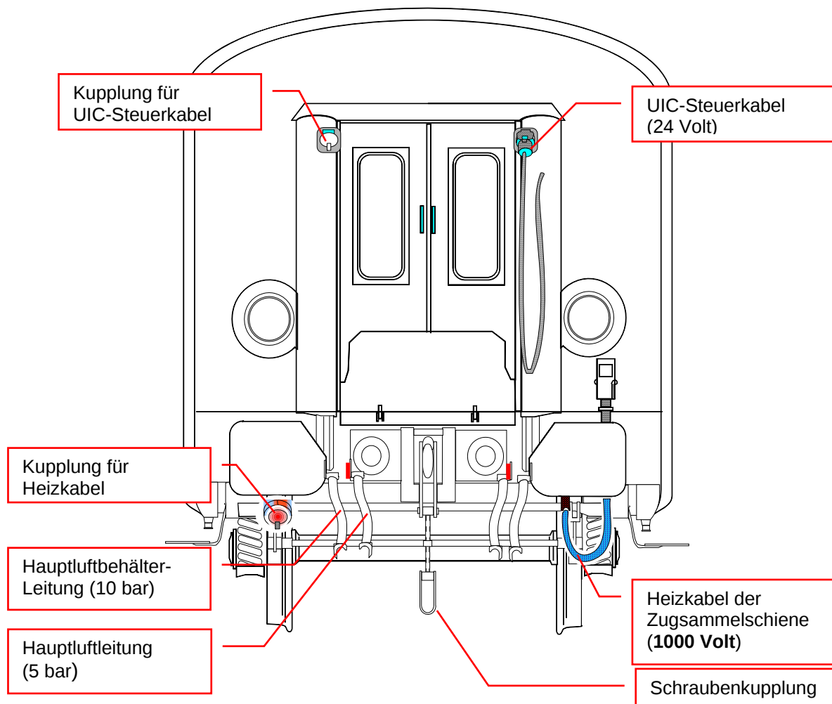
Abbildung 7.07 – Verbindungselemente zwischen Schienenfahrzeugen
