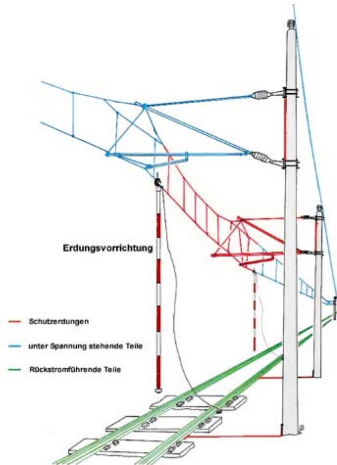
Abbildung 8.10 – Anbringung der Erdungsstangen
