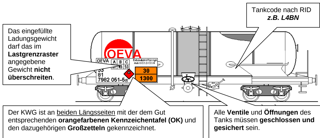
Abbildung 9.02 – Kennzeichnung: Kesselwagen mit Gefahrgut
